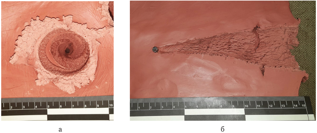
Рис. 19. Характер пошкодження балістичного пластиліну після влучання досліджуваного уражаючого елемента за контактної швидкості 648,3 м/с
