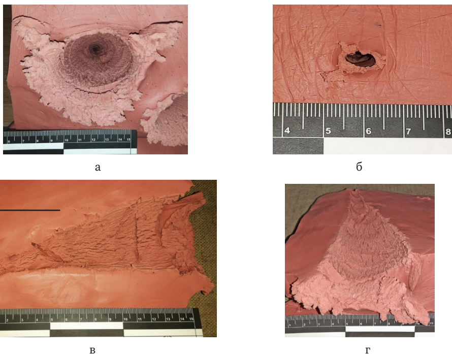
Рис. 30. Загальний вигляд вхідного отвору (а), вихідного отвору (б) і каналу пошкодження (в, г), завданого влучанням уражаючого елемента за контактної швидкості 770,4 м/с (напрямок руху уражаючого елемента позначено стрілкою)
