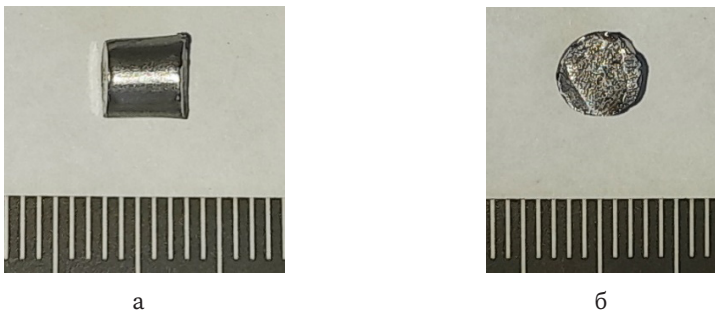
Рис. 21. Загальний вигляд готового уражаючого елемента після влучання в блок балістичного пластиліну
