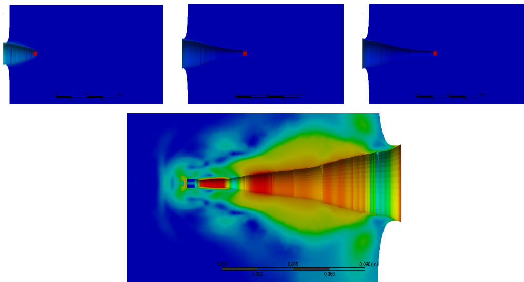
Рис. 34. Результати комп'ютерної симуляції процесу формування каналу пошкодження, завданого циліндричним уражаючим елементом, отримані проф. О. Ларіним під час досліджень 12
