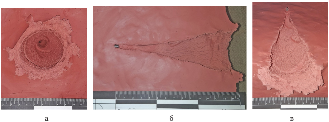
Рис. 20. Характер пошкодження балістичного пластиліну після влучання досліджуваного уражаючого елемента за контактної швидкості 712,3 м/с
