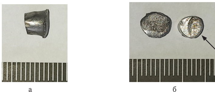
Рис. 23. Загальний вигляд готового уражаючого елеента після влучання в блок балістичного пластиліну та порівняння його із недеформованим зразком (позначено стрілкою)
