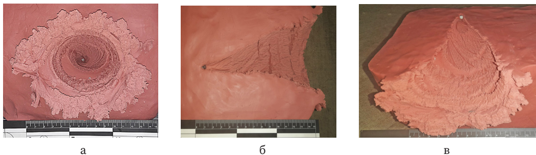
Рис. 24. Характер пошкодження балістичного пластиліну після влучання досліджуваного уражаючого елеента за контактної швидкості 975,6 м/с
