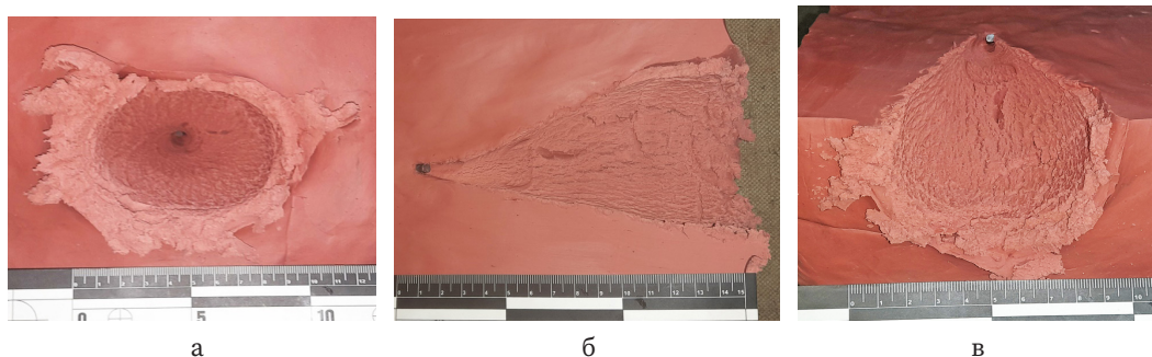
Рис. 22. Характер пошкодження балістичного пластиліну після влучання досліджуваного уражаючого елеента за контактної швидкості 963,2 м/с
