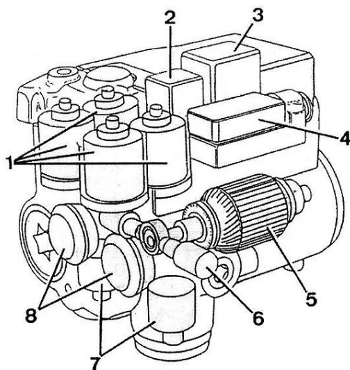
Рис. 2. Електрогідравлічний модулятор: 1 — електромагнітні клапани, 2 — реле гідронасоса, 3 — реле електромагнітних клапанів, 4 — електричний роз'єм, 5 — електродвигун електронасоса, 6 — поршневий елемент насоса, 7 — акумулятор тиску, 8 — глушник
