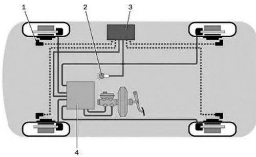
Рис. 1. Принципова схема ABS легкового автомобіля: 1 — датчик швидкості обертання коліс, 2 — сигнальна лампа, 3 — електронний блок управління (ECU), 4 — виконавчі пристрої
